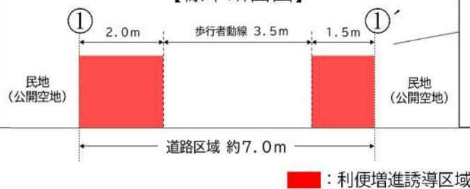
【標準断面図】
