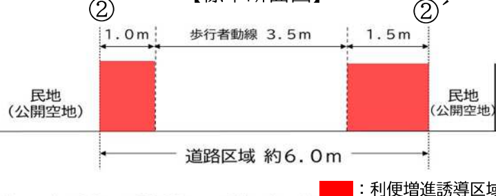
【標準断面図】
