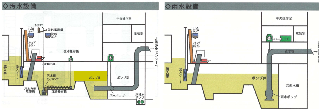
ポンプ場イメージ図
