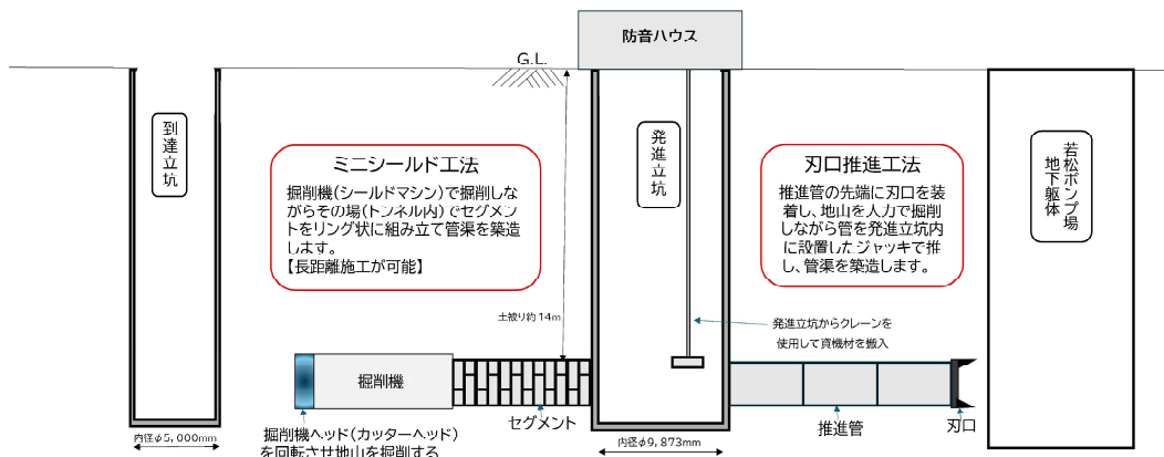
管渠築造工事イメージ図
