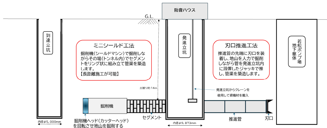
管渠築造工事イメージ図
