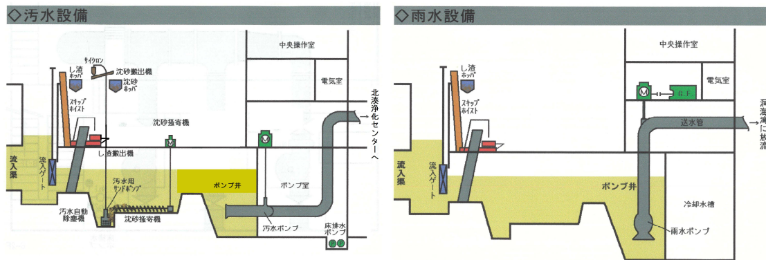
ポンプ場イメージ図
