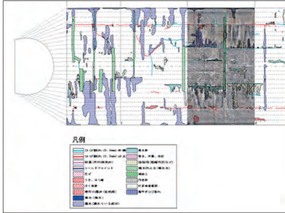
MIMM画像計測解析結果(変状展開図)
