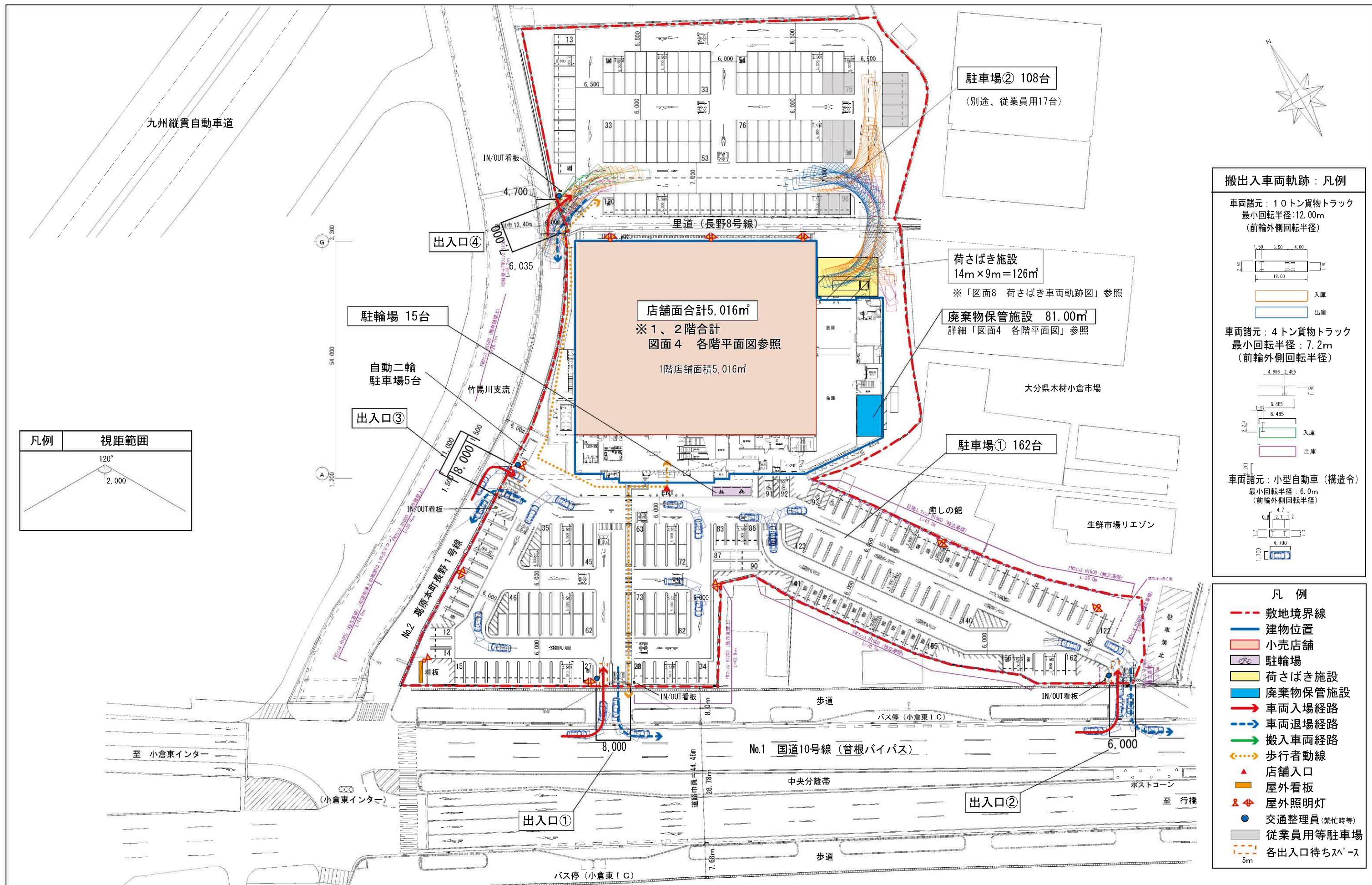
図面 3 建物配置図兼 1 階平面図 (S=1/800)
