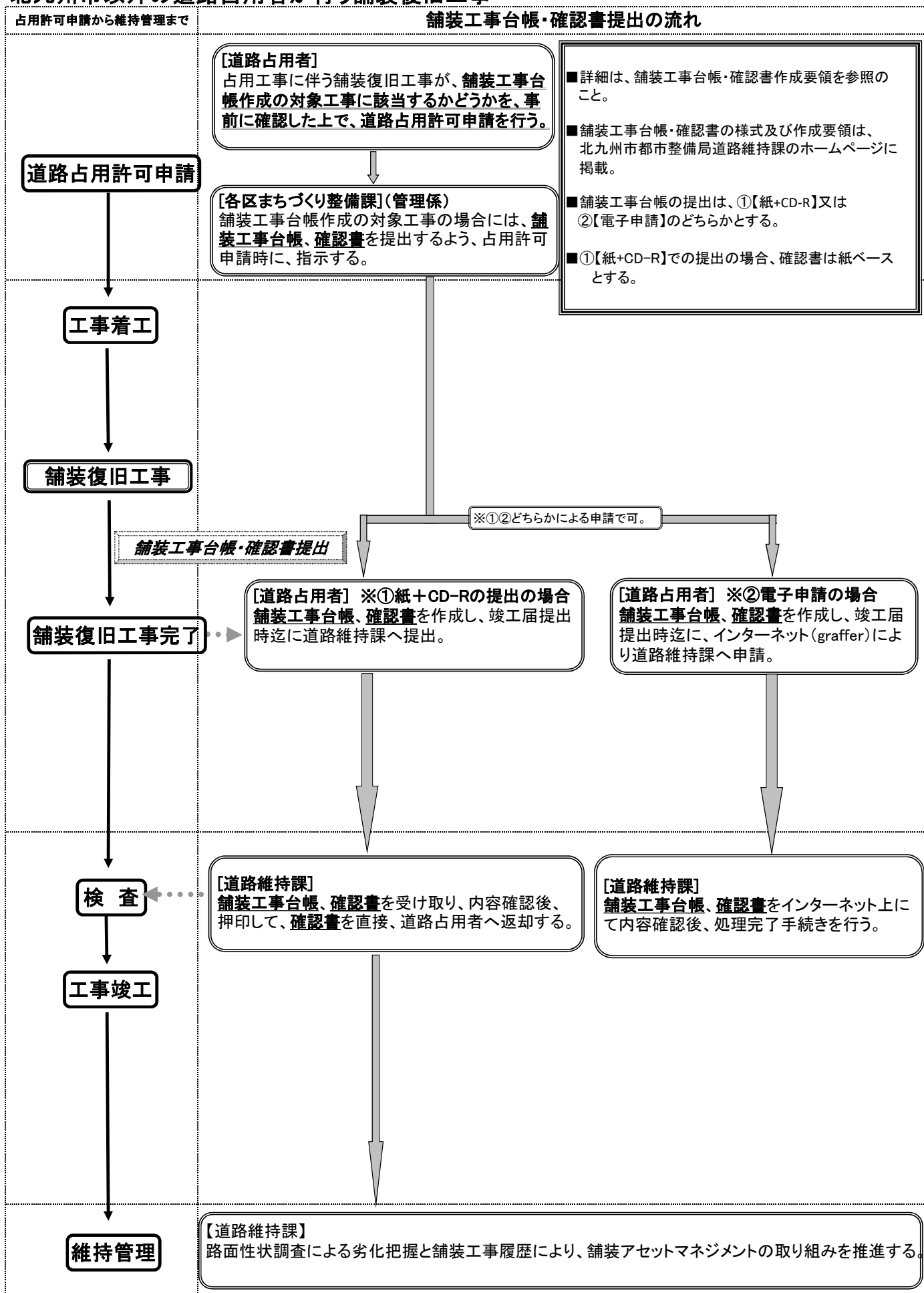
図 6.1 舗装工事台帳・確認書、作成・収集フロー
