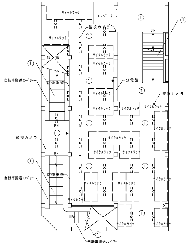
2階平面図 S=1:200
