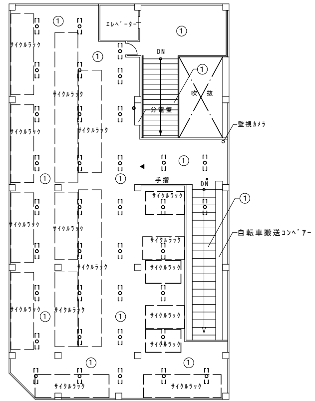
4階平面図 S=1:200
