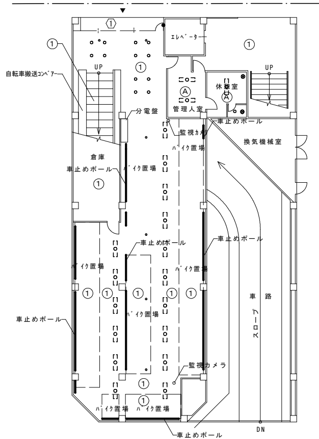
1階平面図 S=1:200
