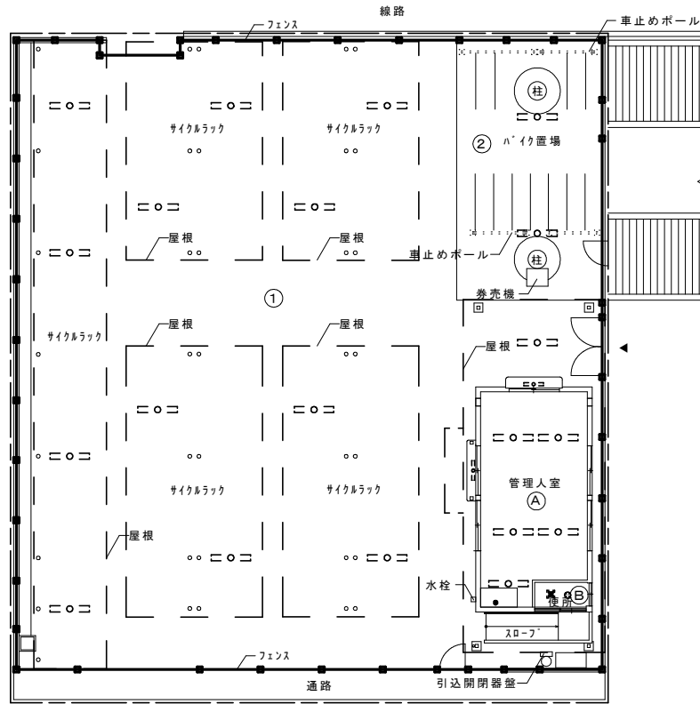
平面図 S=1:150
