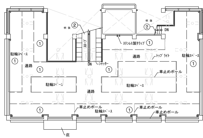
2階平面図 S=1:200
