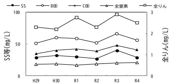
図-2 初沈流出水の経年変化
