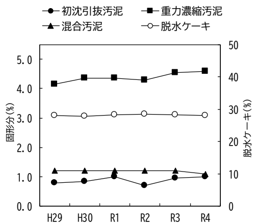
図-6 汚泥の固形分の経年変化
