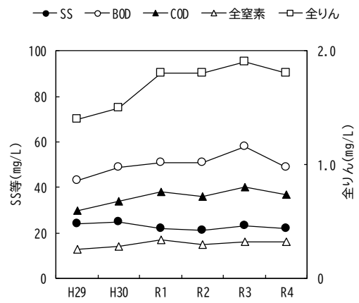
図-2 初沈流出水の経年変化
