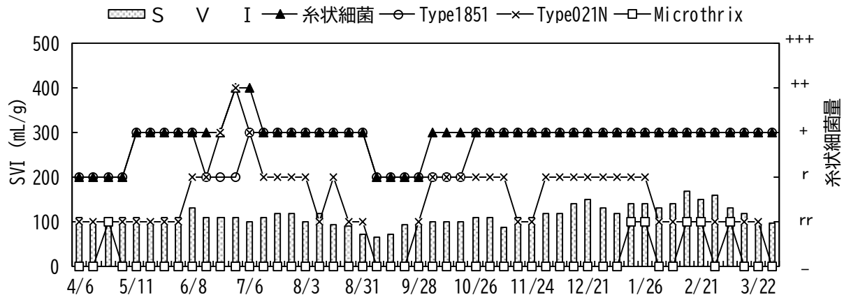
図-7 反応タンク混合液(標準槽)のSVIと糸状細菌
