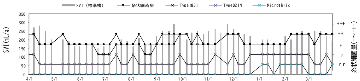
図-7 反応タンク混合液(標準槽)のSVIと糸状細菌
