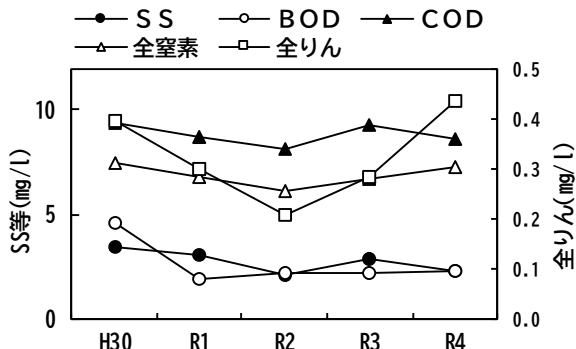
図-5 処理水(深槽)の経年変化
