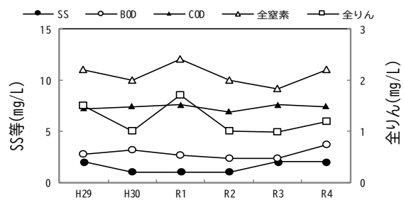
図-5 深槽処理水の経年変化
