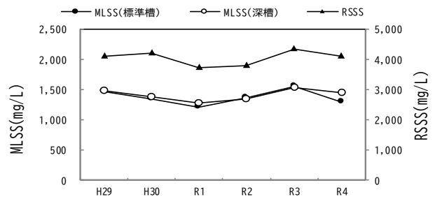
図-6 MLSS等経年変化
