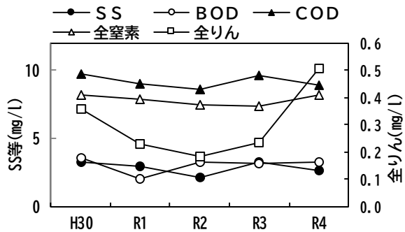
図-4 処理水(標準槽)の経年変化
