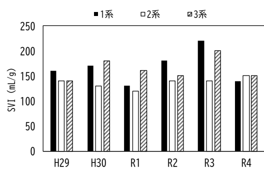
図-7 SVIの経年変化
