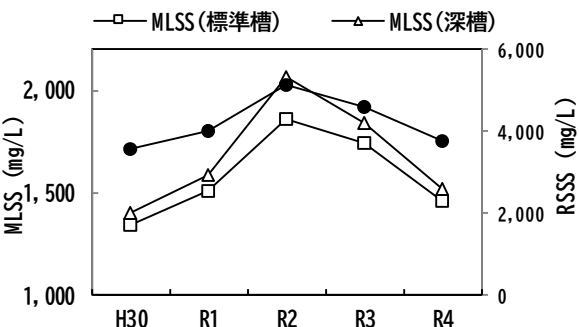
図-6 MLSS等の経年変化
