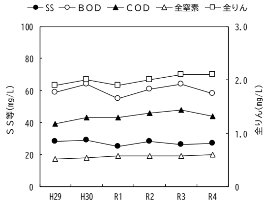
図-2 初沈流出水の経年変化
