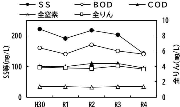
図-1 処理場流入水の経年変化
