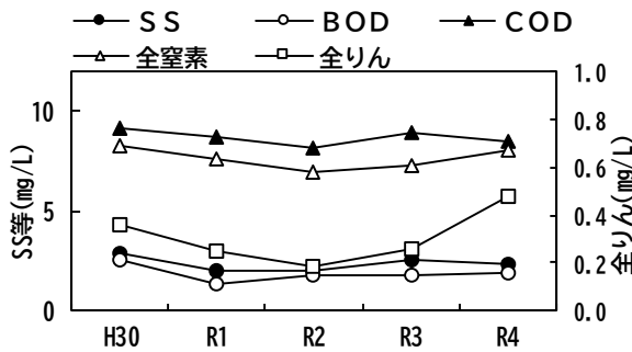
図-3 放流水の経年変化
