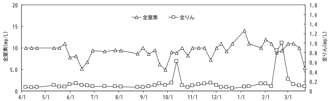
図-4 放流水中の全窒素と全りんの濃度変化
