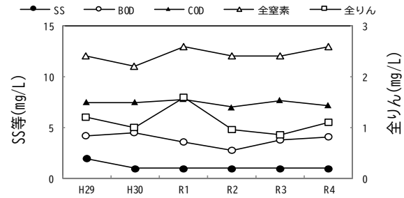
図-4 標準槽処理水の経年変化
