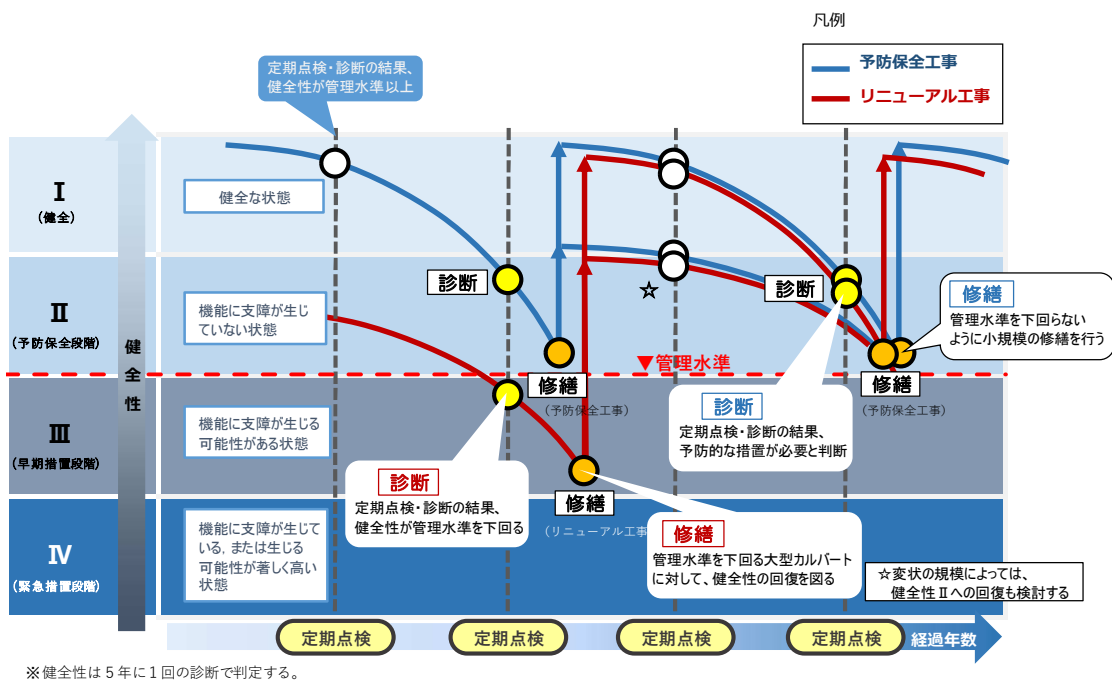
図 4.1 予防保全工事とリニューアル工事の概念図
