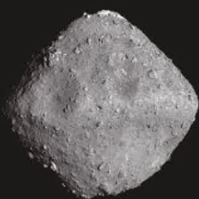
小惑星リュウグウ ©JAXA、東大など
