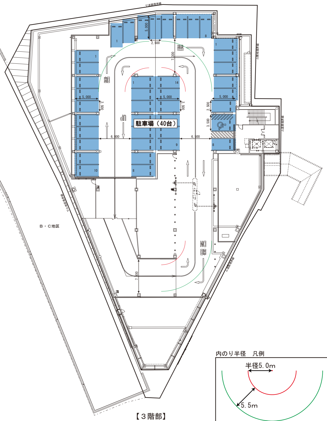
資料-4.1 2階・3階平面図
