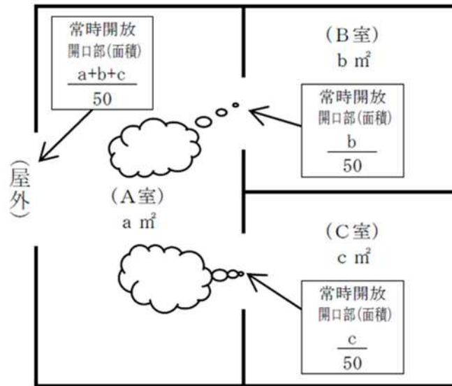
(同一区画としてみなすことができる例)
