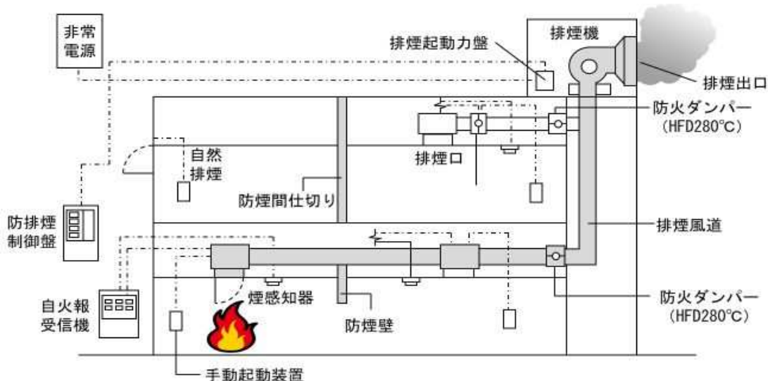
【消火活動拠点以外の機械排煙方式の概要図】
