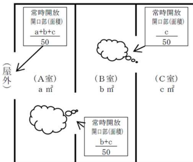
(同一区画としてみなすことができない例) ※C室がB室を介しているため。
