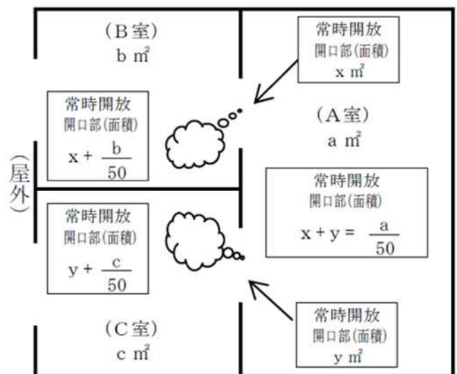
(同一区画としてみなすことはできない例) ※A室の開放がxとyの2面開放となっているため。
