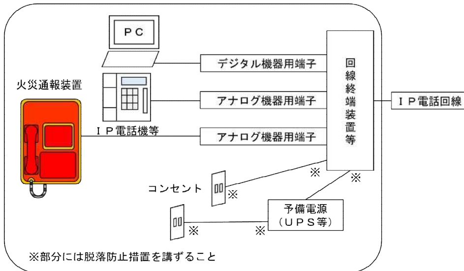
第15-6図 IP電話回線における火災通報装置の接続部分について
