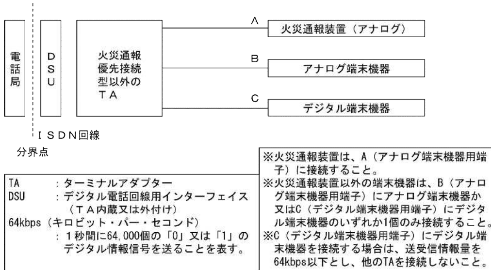
第15-11図 火災通報優先接続型TA以外のTAを用いた接続例
