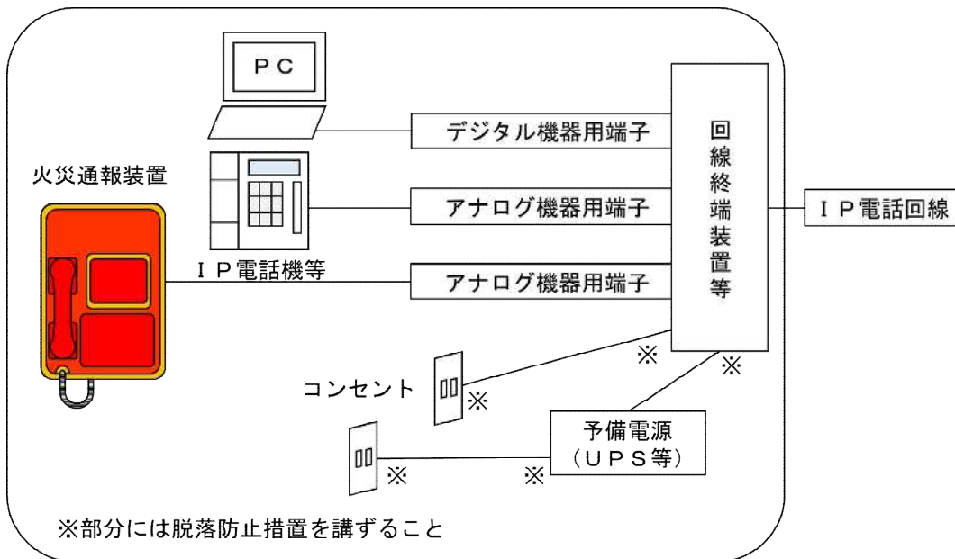
第15-7図 回線終端装置等に複数のアナログ端末機器接続用端子がある場合
