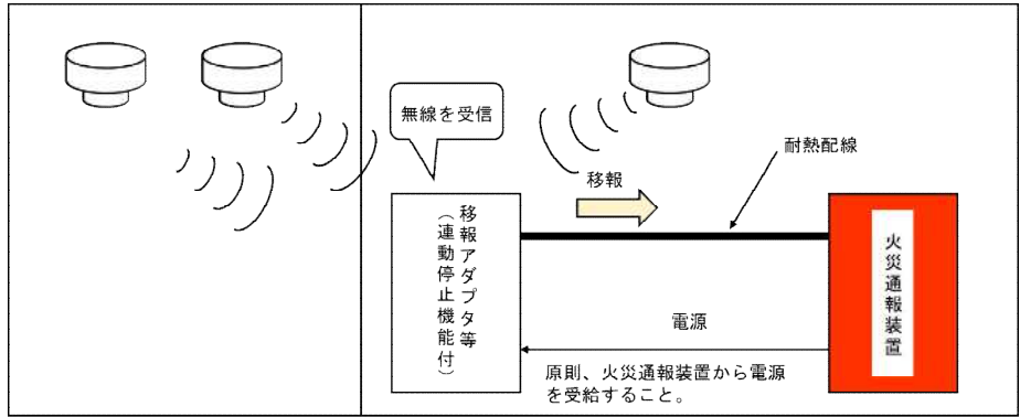
第 15-14 図 火災信号を無線で受信する場合
