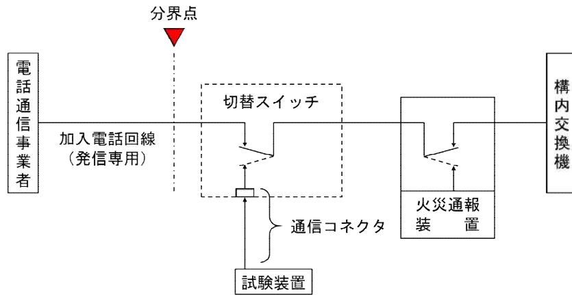
第15-3図 分界点を通信コネクタ以外の方法とする場合
