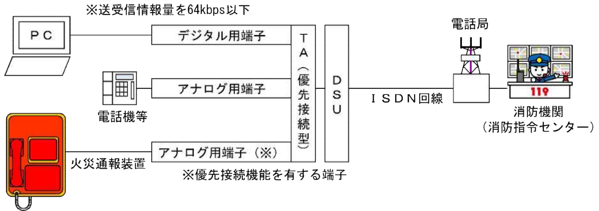
第 15-9 図 I S D N回線に接続する火災通報装置の概要図
