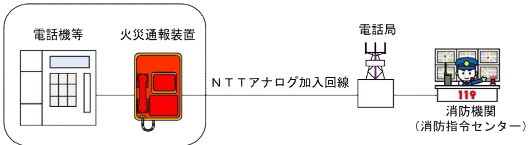
第 15-2 図 専用回線以外で接続する火災通報装置の概要図
