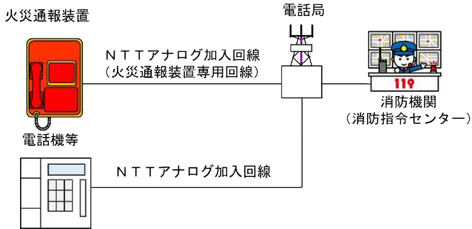
第 15-1 図 NTT 電話回線に専用回線で接続する火災通報装置の概要図
