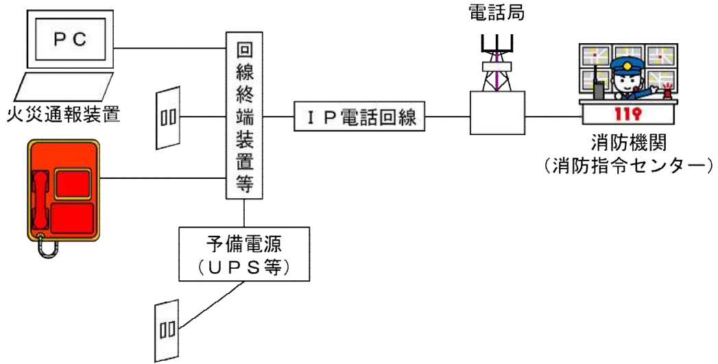
第15-5図 IP電話回線に接続する火災通報装置の概要図
