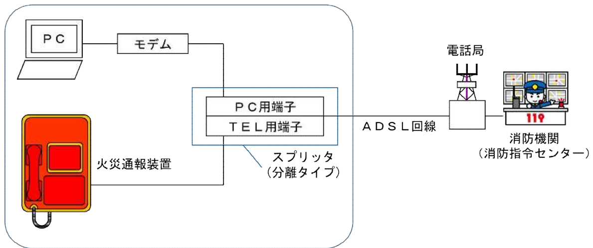
第 15-8 図 ADSL回線に接続する火災通報装置の概要図
