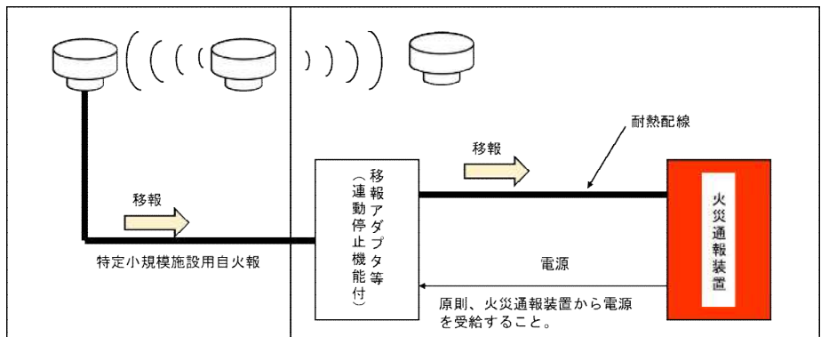
第 15-15 図 火災信号を有線で受信する場合
