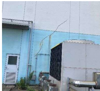
外壁亀裂
