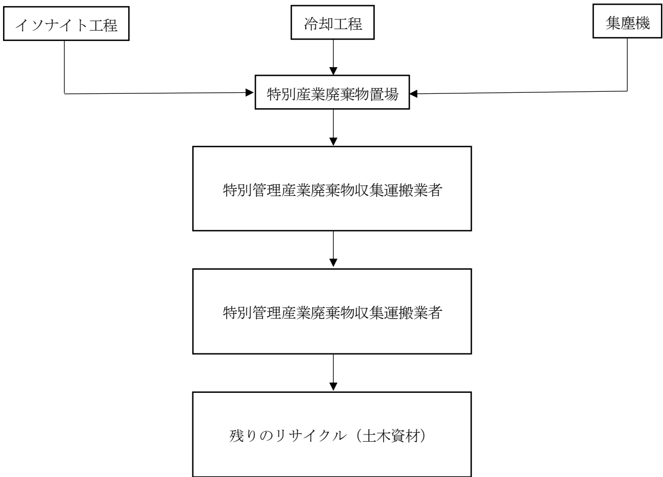
図2. 汚泥処理フローシート
