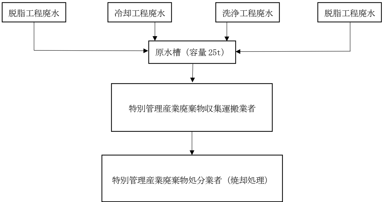
図1. 廃水処理フローシート
