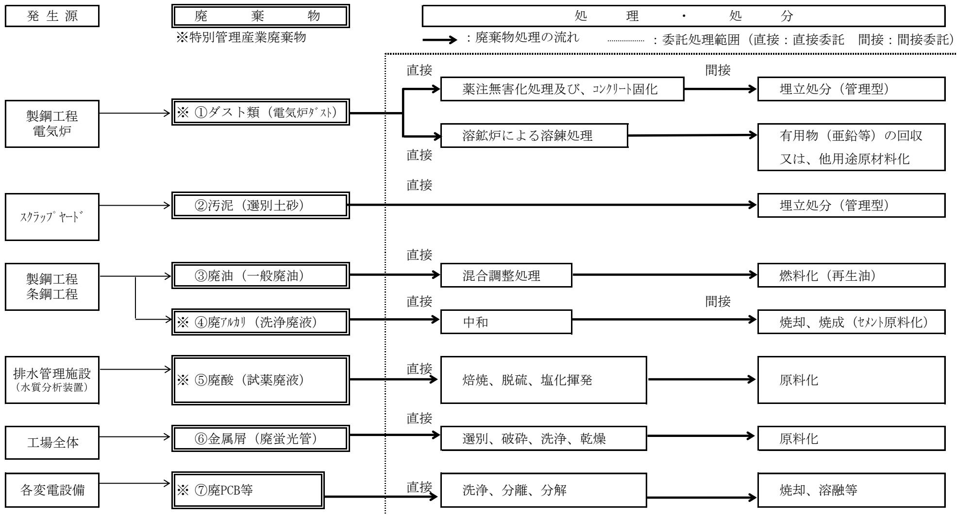
図1. 廃棄物処理フロー図
