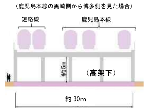
折尾駅高架下 断面図 (A)
