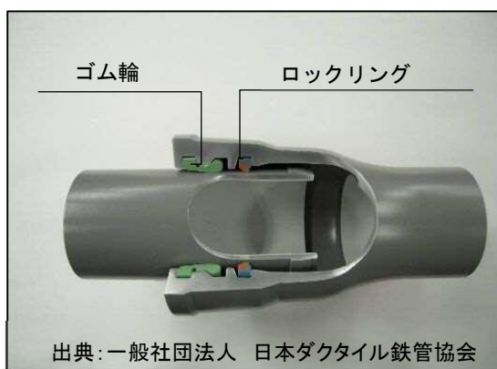
耐震継手 GX 形ダクタイル鋳鉄管
