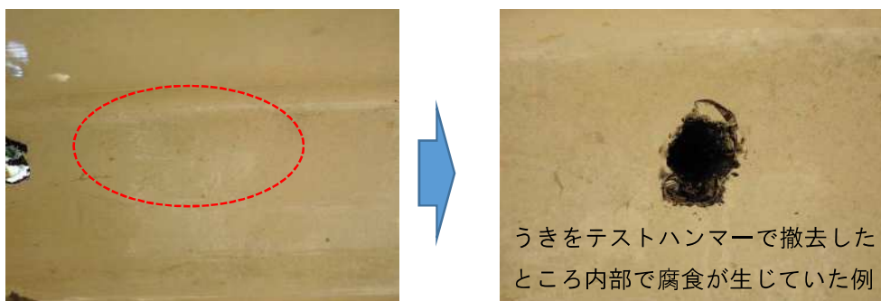
塗装片を取り除いた状態の例（床版）
